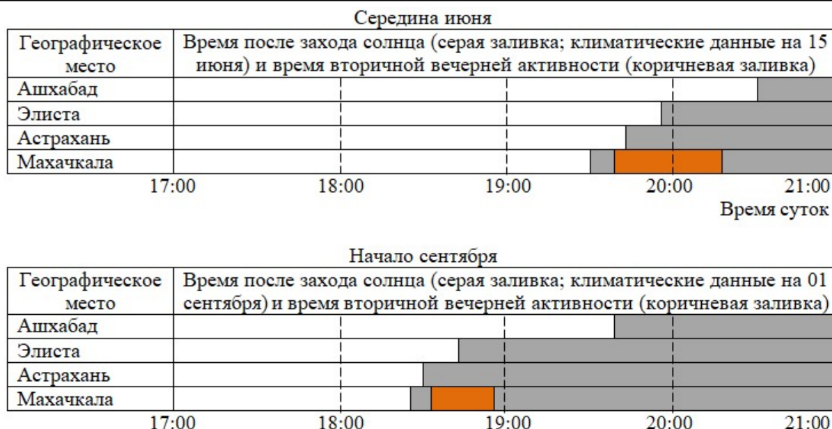
Рис. 8. Время захода солнца и проявлений вторичной вечерней активности в разных регионах, населенных ушастыми круглоголовками Fig. 8. Time of sunset and manifestations of secondary evening activity in different regions inhabited by toad-headed agamas
