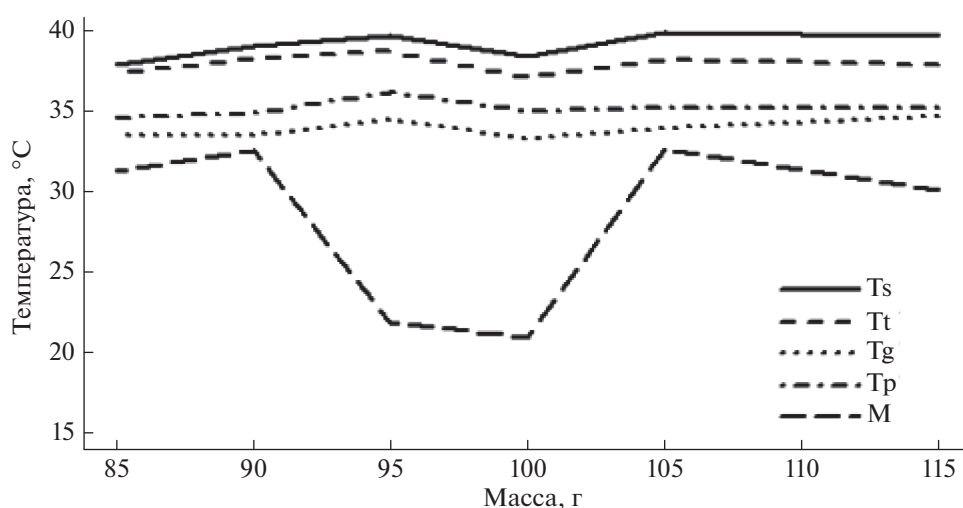
Рис. 3. Соотношение оценок температуры тела у гадюк разного размера ( T_s — высшая максимальная, T_t — типичная максимальная, T_g — добровольная максимальная, T_p — средняя пиковая максимальная, M — средняя температура тела за день).
