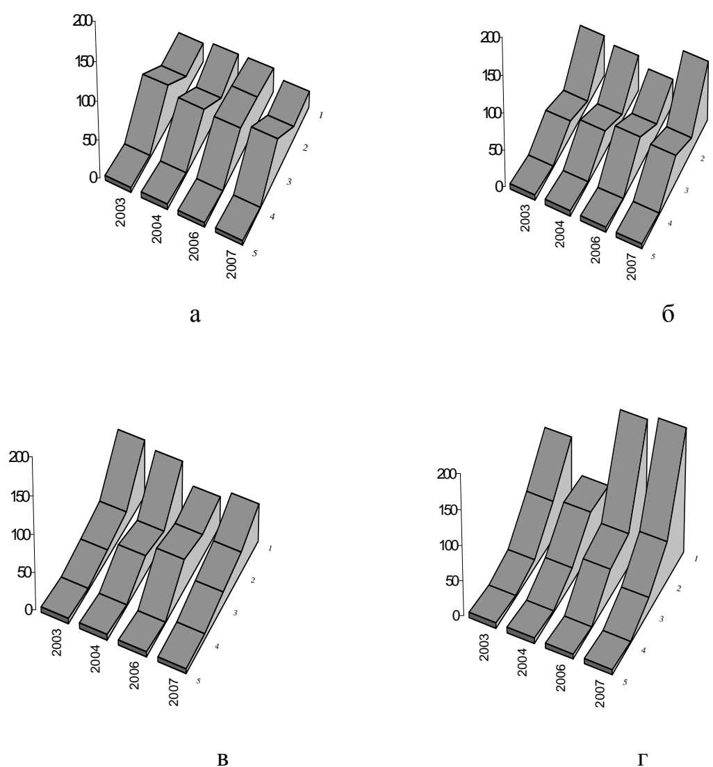
Рисунок 2 - Гидрохимические показатели нерестовых водоемов за ряд лет (а - многоэтажная застройка, б - малоэтажная застройка, в - лесопарк, г – загородная популяция; 1 – сульфаты, мг/дм 3 ; 2 – хлориды, мг/дм 3 ; 3 – перманганатная окисляемость, мг/дм 3 ; 4 - БПК-5, мг/дм 3 ; 5 - рН)
