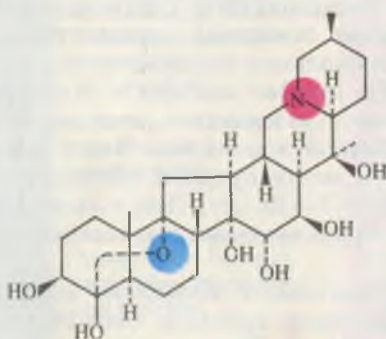
зигаденин
