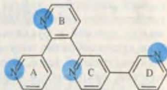
немертиллен
