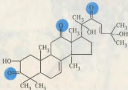
элатерин А
