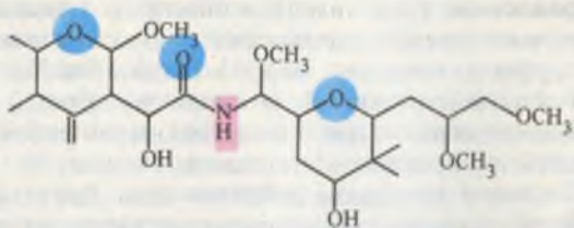
педерин
