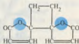
анемонин
