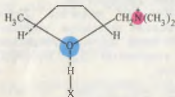
мускарин
