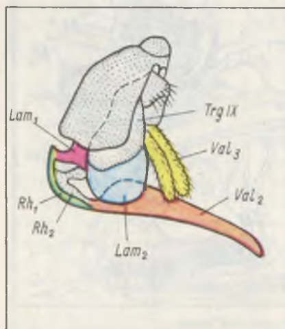
Рис. 29. Строение жалящего аппарата осы. Обозначения см. рис. 27 и 28
