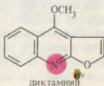
диктамнин
