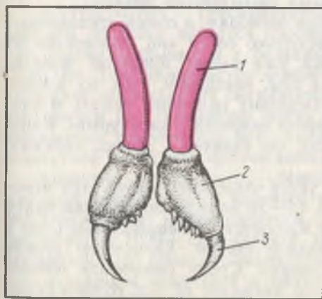
Рис. 22. Ядовитый аппарат тарантула:
