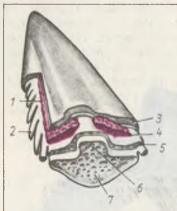
Рис. 50. Схема строения шипа ската-хвостокла:
