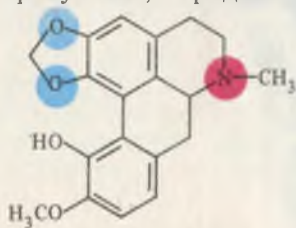
бульбокапнин
