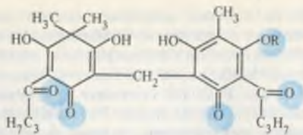
флаваспидиновая кислота R=H
