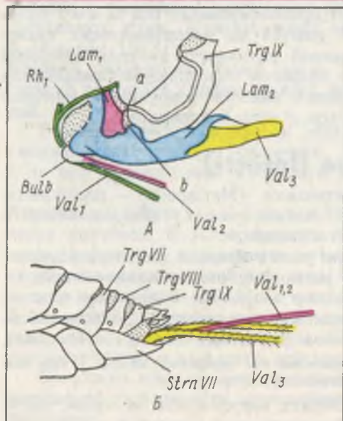
Рис. 27. Строение жалящего аппарата наездников:
