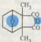
кантаридин
