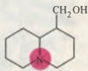
лупинин
