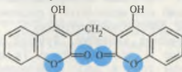
дикумарин
