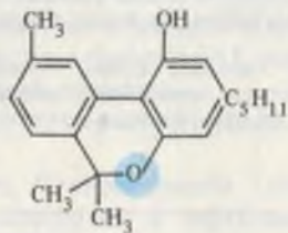
каннабинол
