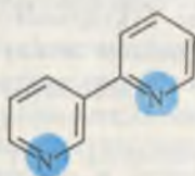
2,3'-бипиридил
