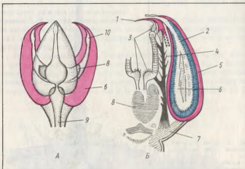
Рис. 15. Ядовитая глобиферная педицилляррия морского ежа (А) и схема ее строения (Б):
