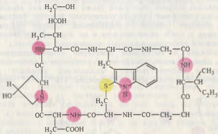
аманин
