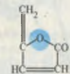
протоанемонин
