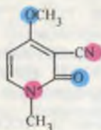
рицинин
