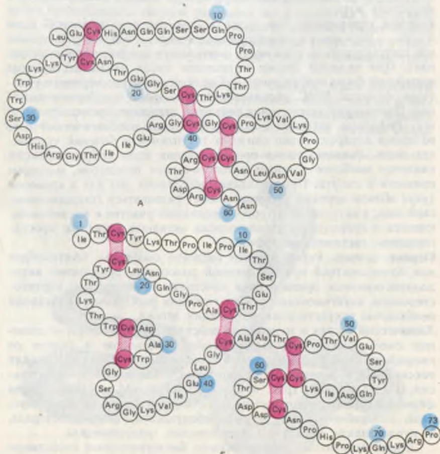
Рис. 66. Первичная структура нейротоксина II (А) и нейротоксина I (Б) из среднеазиатской кобры
