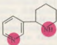
анабазин
