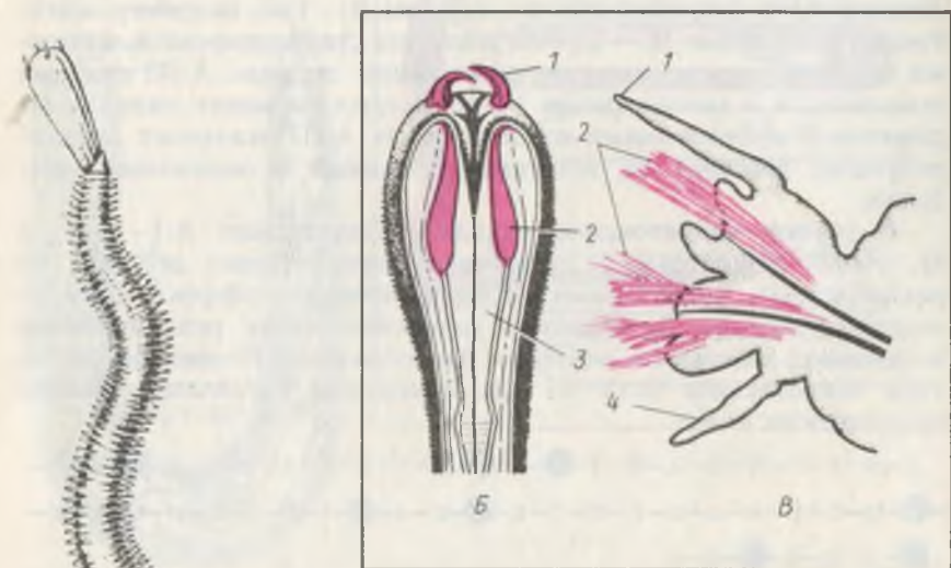
Рис. 7. Строение ядовитого аппарата многощетинкового червя:
