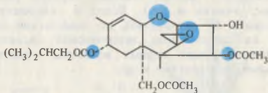
Т-2-токсин
