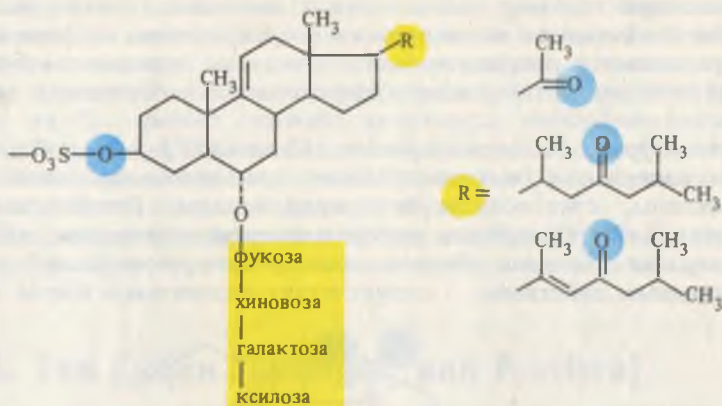
астеросапонин В
