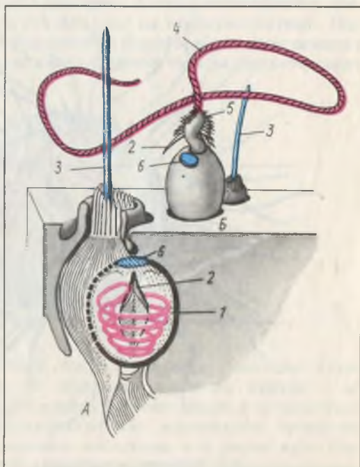
Рис. 1. Строение стрекательной клетки (книдобласта) кишечнополостных впокоящемся состоянии (А) и с выброшенной стрекательной нитью (В): 1 — нематоциста; 2 — стилет; 3 — книдоциль; 4 — стрекательная нить; 5 — шипы; 6 — крышечка
