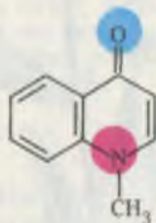
эхинопсин
