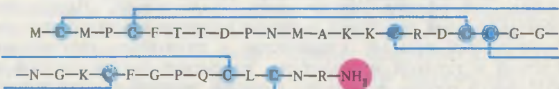
инсектотоксин И 2
