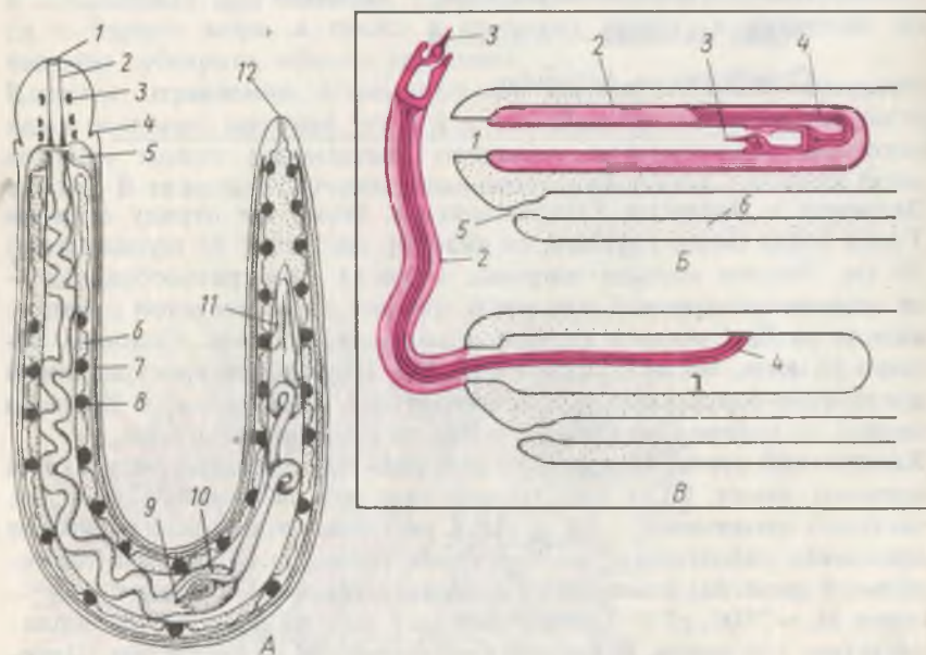
Рис. 6. Схема строения вооруженной немертины (А) и ее ядовитого аппарата (Б и В):
