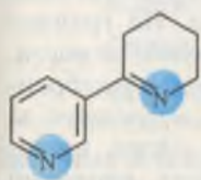
Анабазеин
