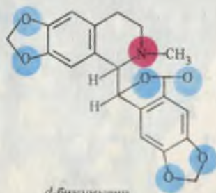
d-бикукулин
